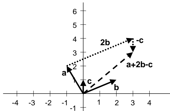
Abbildung 1: Vektoren \mathbf{a} , \mathbf{b} , \mathbf{c} sowie \mathbf{a} + 2\mathbf{b} - \mathbf{c}
