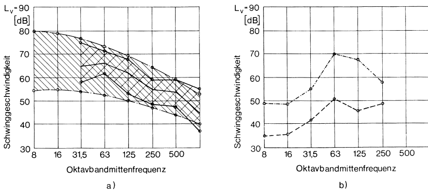
Bild 5.6. Schwinggeschwindigkeitsspektren an der Tunnelwand als Eingabegröße für (5.2) mit v_{\text{ref}} = 5 \cdot 10^{-5} \text{ mm/s}
