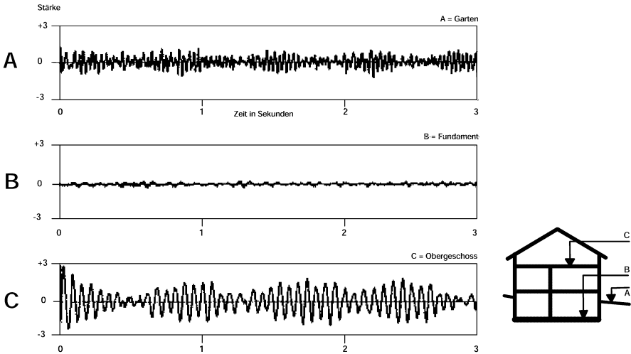
Bild 5.12. Gemessene Erschütterungsübertragung in einem Gebäude A: Garten, B: Fundament, C: Obergeschoss
