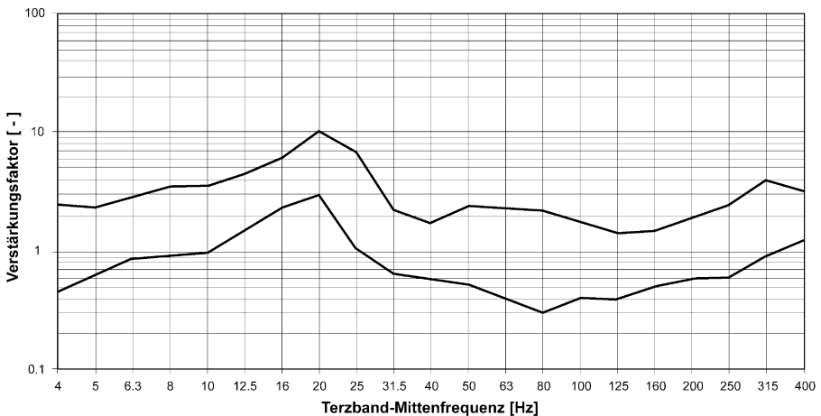
Bild 5.9. Übertragungsspektren vom Boden auf die-Geschossdecken. Klar erkennbar ist, dass im Bereich der Eigenfrequenz der Decken (20Hz) die Spektralamplituden stark angehoben sind (Resonanzeffekte). (Rutishauser, 2004)
