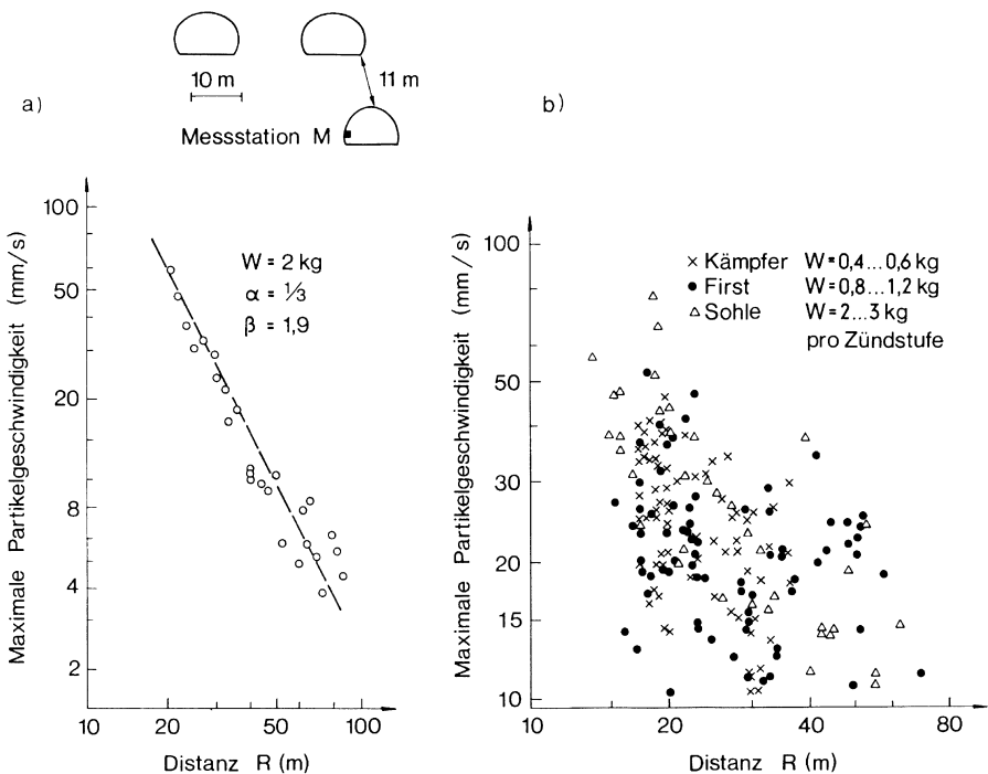
Bild 5.10. Sprengerschütterungen (nach Studer und Süssstrunk, 1981); a) Resultate einer einzelnen Messstation M; Fels: Gneis, Ausbruch des Profils; b) Daten von verschiedenen Messstationen in verschiedenen Tunnelquerschnitten
