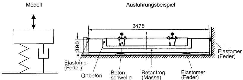
Bild 5.18. Feder Masse-System
