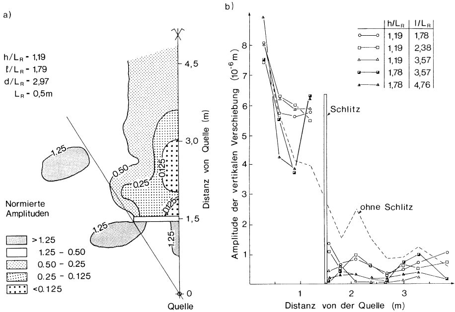
Bild 5.20. Abschirmwirkung von offenen Schlitzen; a Normierte Amplituden, h = Schlittiefe, l = Schlittlänge, d = Distanz von der Quelle, L_R = Rayleighwellenlänge; b Vertikale Verschiebungsamplituden in Abhängigkeit der Entfernung (nach Woods, 1968)
