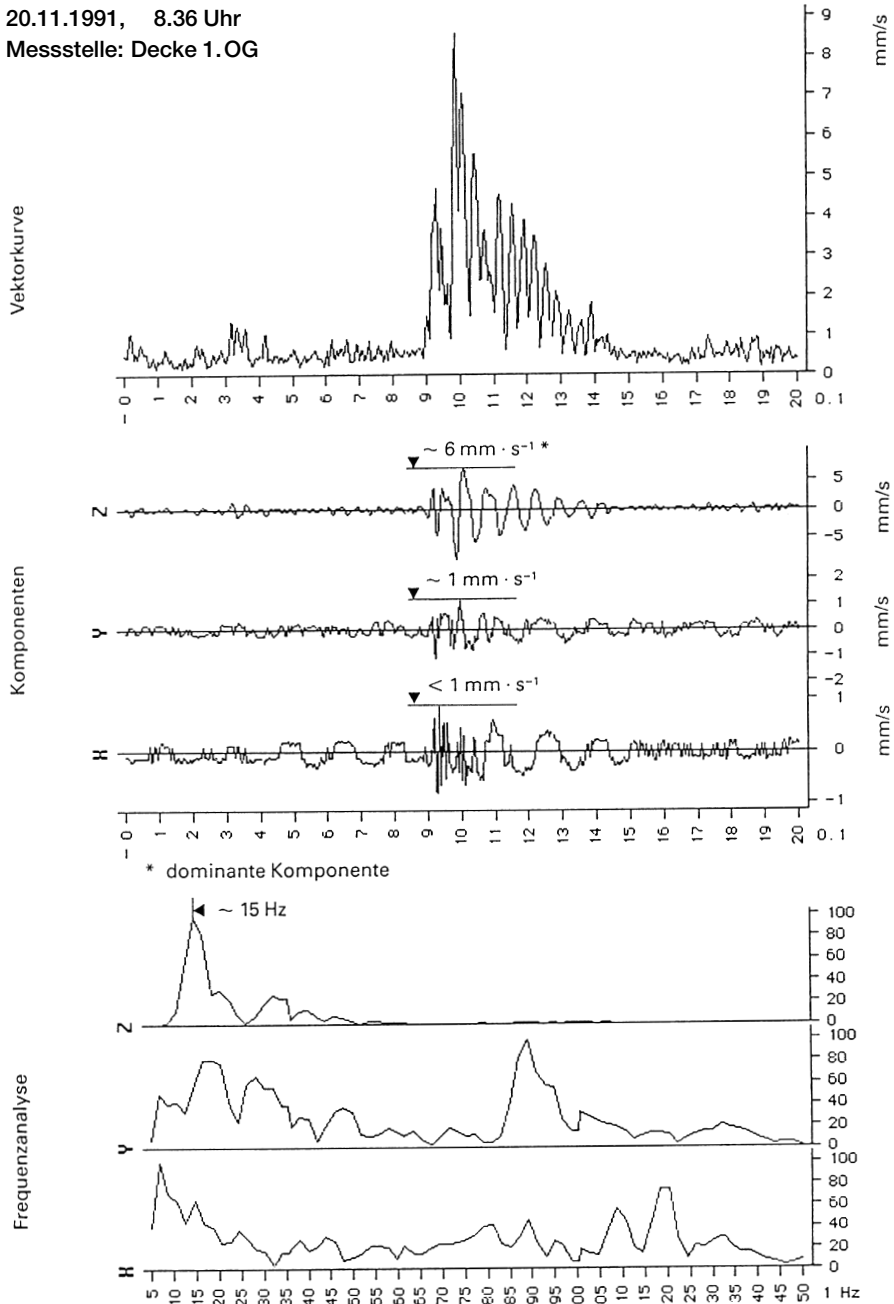
Bild 5.13. Beispiel: Erschütterungsverlauf (dargestellt Vektor v_R , Komponenten Z, Y, X; maßgebend: v_{Rmax} = 8.5 \text{ mm/s} , Z-Komponente hat die tiefste dominante Frequenz, etwa 15 Hz) (aus Norm SN 640312a)
